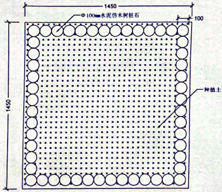
北京中路树池平面图 (水泥仿木树桩)
