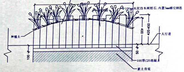
A-A剖面图
